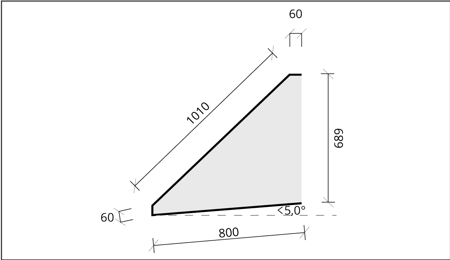
ill. Måsett illustrasjon for montering av baldakin Heavy Duty
