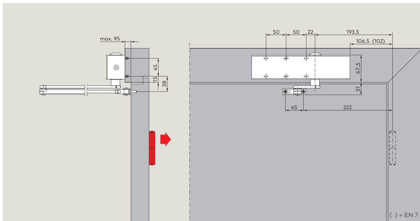
Eksemplet viser venstre (ISO 6) dør; højre (ISO 5) dør spejlvendt
